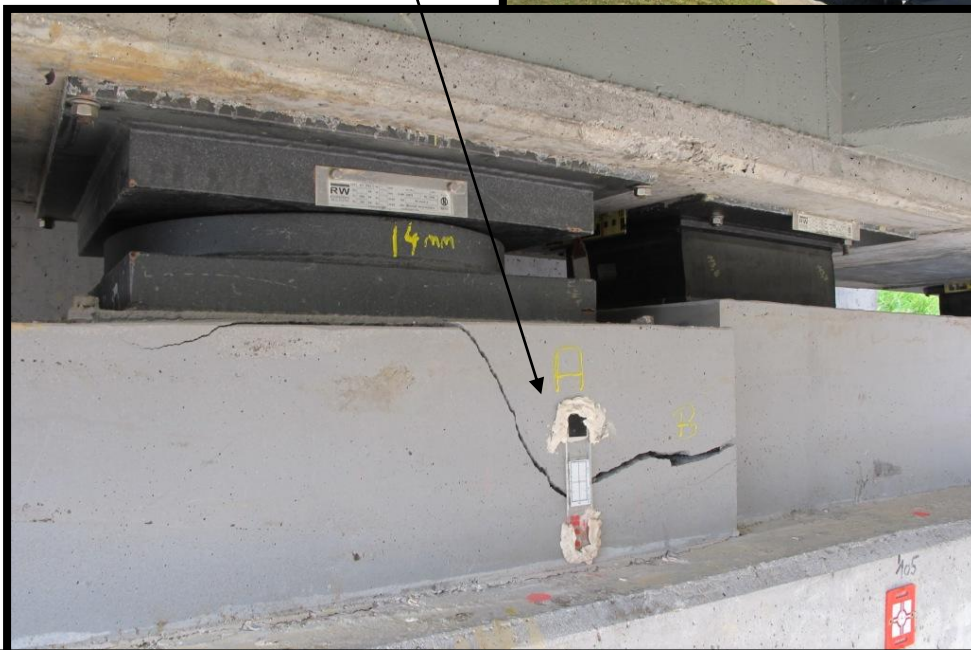
Riss im Brückenaufleger
